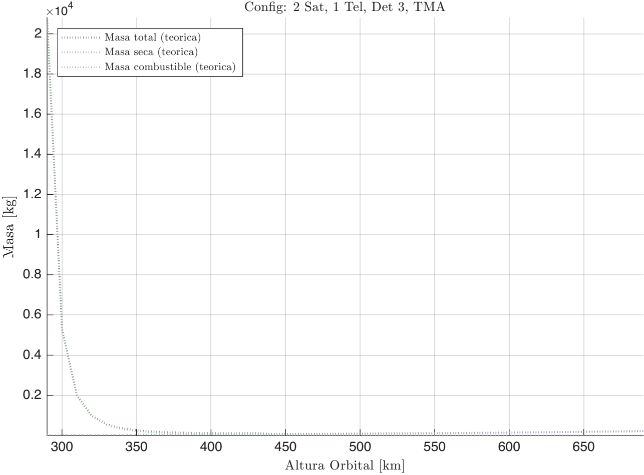
Desglose de Masas vs. Altura Config: 2 Sat, 1 Tel, Det 3, TMA
